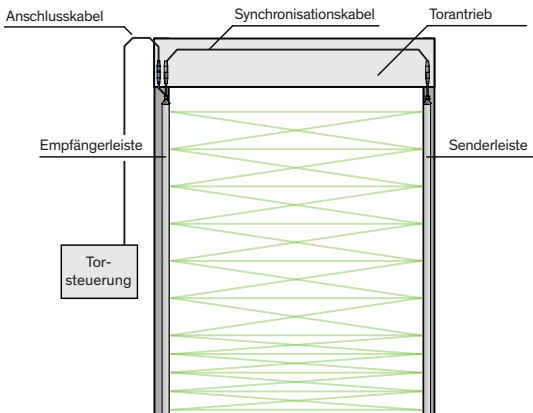
Abb 6: GridScan/Pro Anwendungsübersicht
