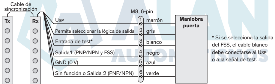
Figura 10: Diagrama de conexión
