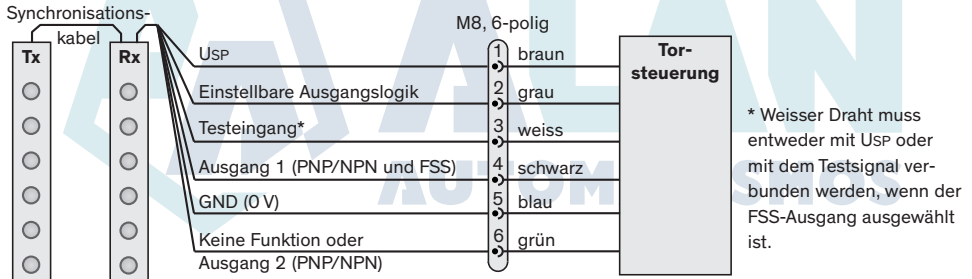
Abb 10: Anschlussdiagramm
